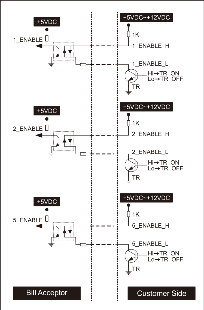
5V Enable Interface-2.
